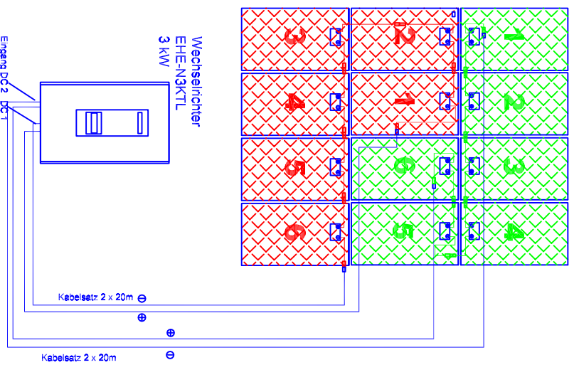
Schrägdach 3 kW
