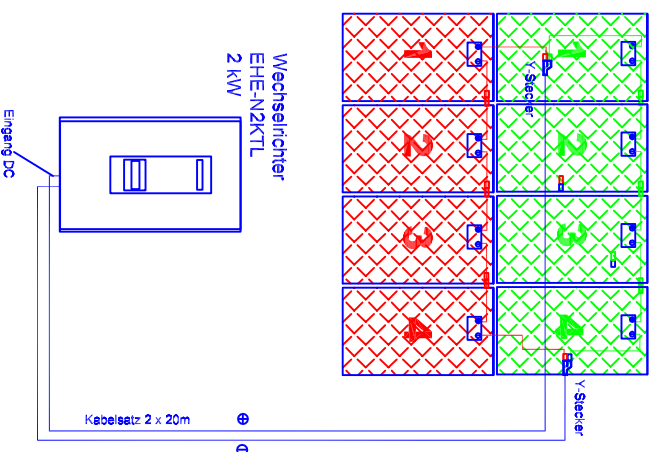
Schrägdach 2 kW
